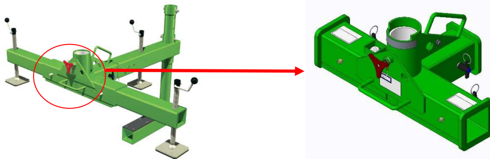
Nachrüstungssatz für Gegengewichtssystem und Mittelteil
