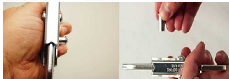
Figure 1 : Le rivet desserré peut s'extraire du crochet.
