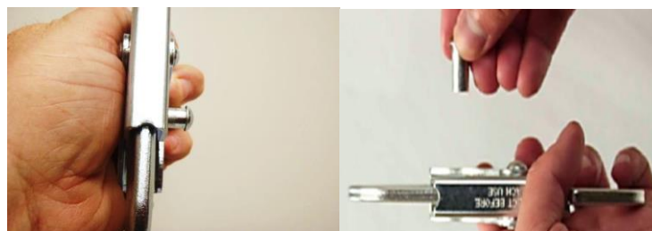
Figure 1 : Un rivet mal serré dépasse du mousqueton.
