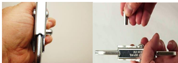
Figura 1: El remache flojo puede sobresalir del gancho.
