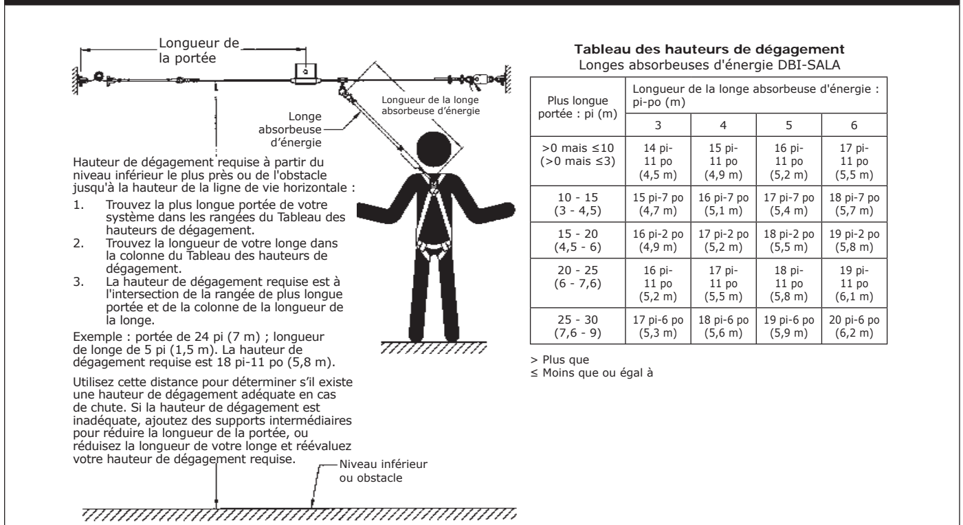
Figure 6 - Exigences en matière de dégagement de la longe absorbeuse d'énergie
